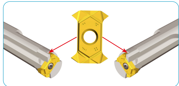
Die neutrale Wendeschneidplatte im Einsatz an linken und rechten Haltern
