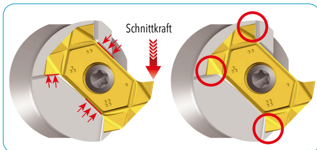
3 Kontaktflächen und Schraubklemmung zum Schutz nicht verwendeter Schneiden
