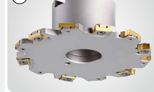
Schlichten des Unterschnitts Finishing undercut
